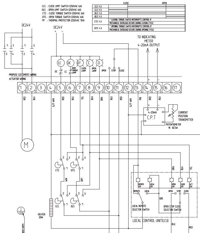
Схема подключения привода на 24 В постоянного тока NA015 - NA028 (LCU, CPT) (NS-87800-C)
