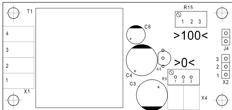
Рисунок А.1 – Плата питания
