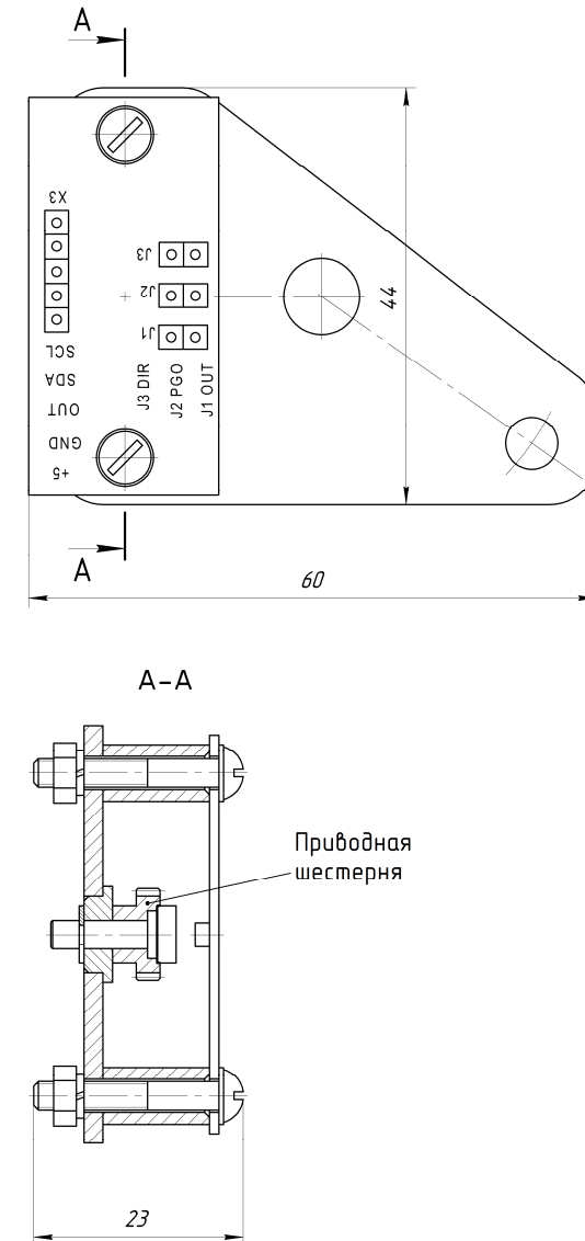
Рисунок А.2 – Плата датчика
