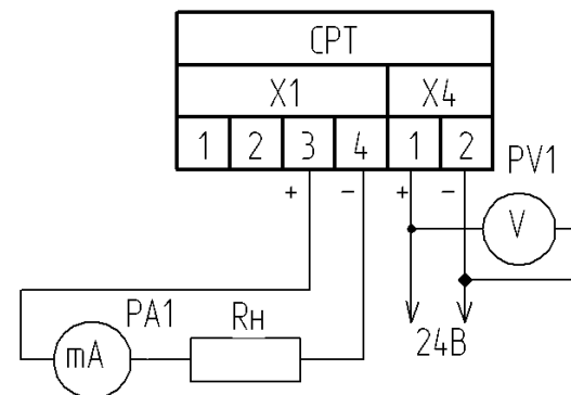
Рисунок В.1 – схема подключения блока, питание 220 В 50 Гц
