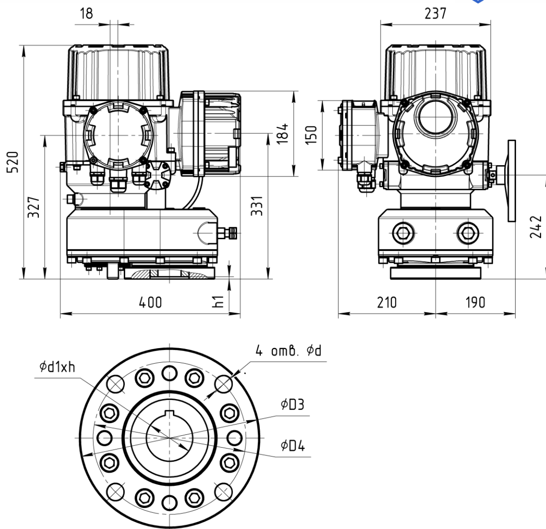
Рис. 2 – Габаритные размеры приводов БИРС 12.5.150...300
