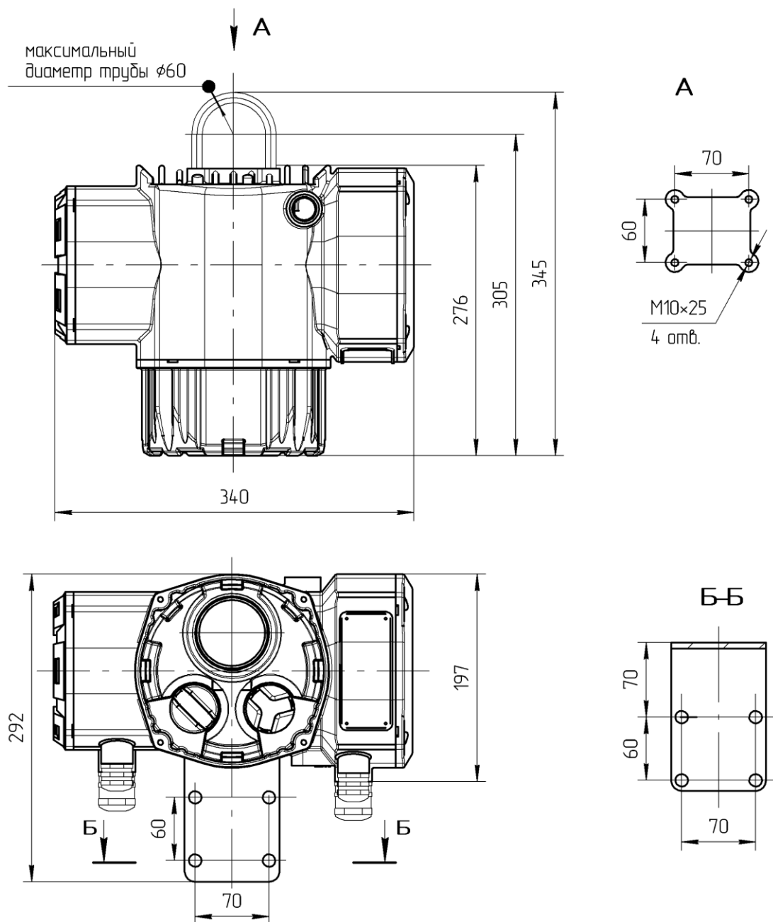
Рис. 3 – Габаритные и присоединительные размеры выносного блока управления
