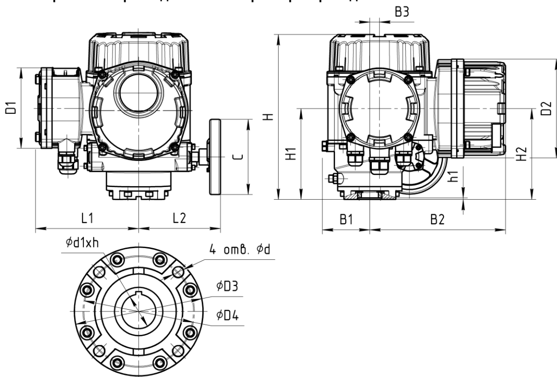
Рис. 1 – Габаритные размеры приводов БИРС 12.5.005...100
