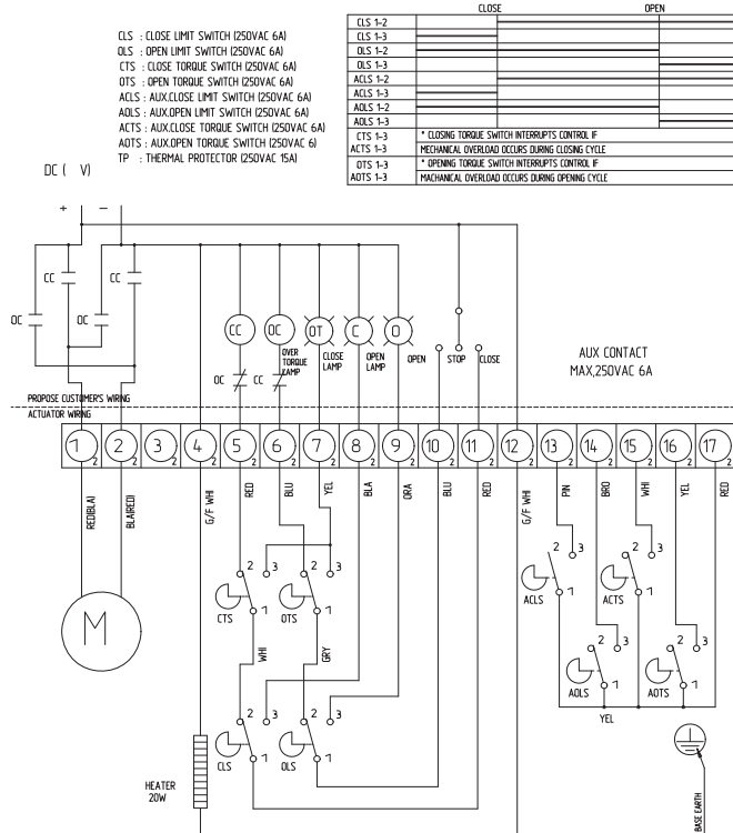
Схема подключения привода на 24 В постоянного тока NA015 - NA028 (ALC, ATC) (NS-82900-C)
