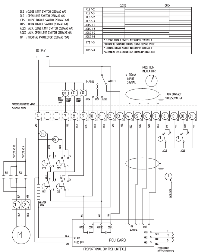
Схема подключения привода на 24 В постоянного тока NA015 - NA028 (ALC, PCU) (NS-82500-C)
