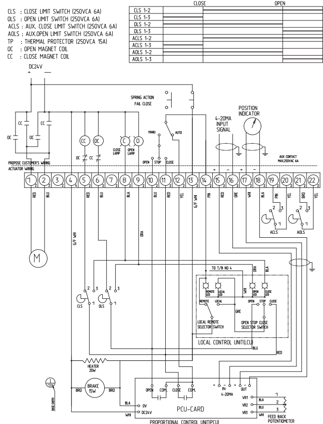
Схема подключения привода на 24 В постоянного тока (ALS, PCU, LCU) (RUC-8257-A)
