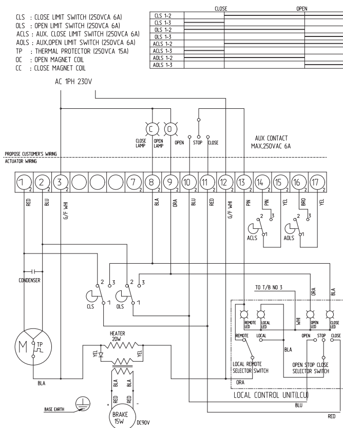
Схема подключения однофазного привода (ALC, LCU) (RUC-2270-A)
