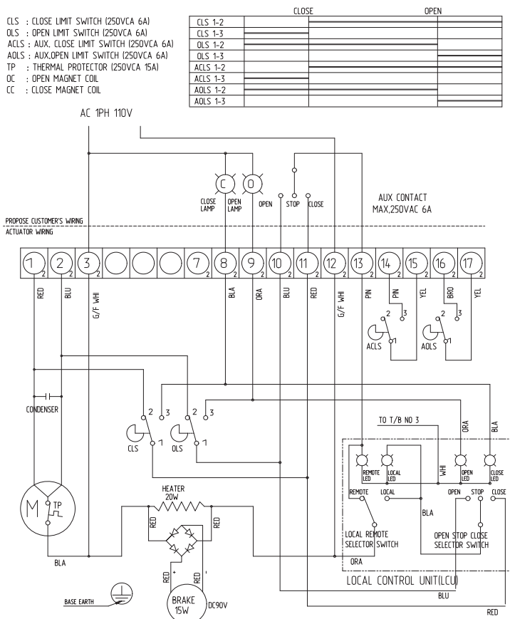
Схема подключения однофазного привода (ALC, LCU) (RUC-1270-A)
